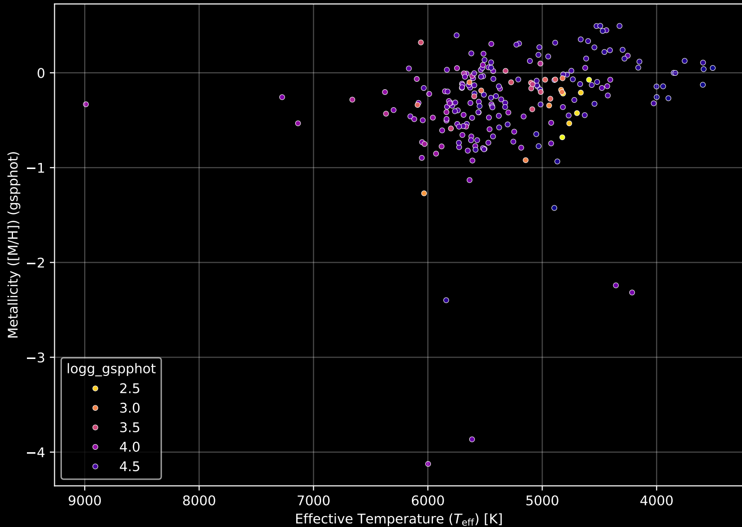
APOGEE DR17 Field: [133-55-O] Stellar Population Parameters (n= 214)
